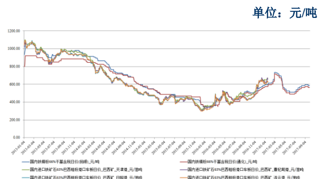
图 4：近年来国内外铁精粉价格走势情况
